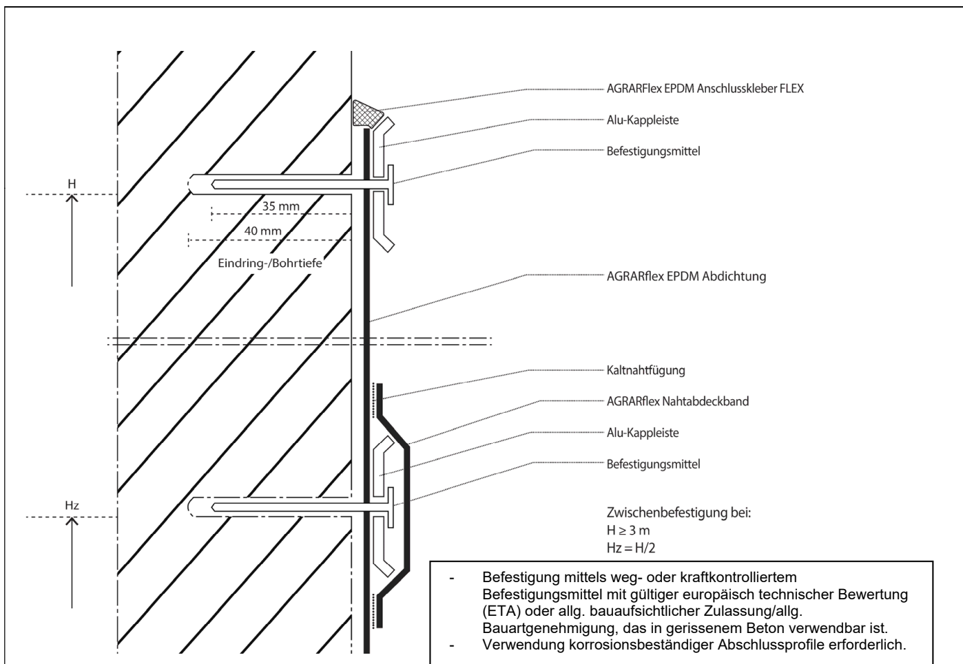
Abb. 1: Ausbildung der oberen Befestigung an der Wand (30 cm über OK Gelände) (oben) und Zwischenbefestigung (unten)
