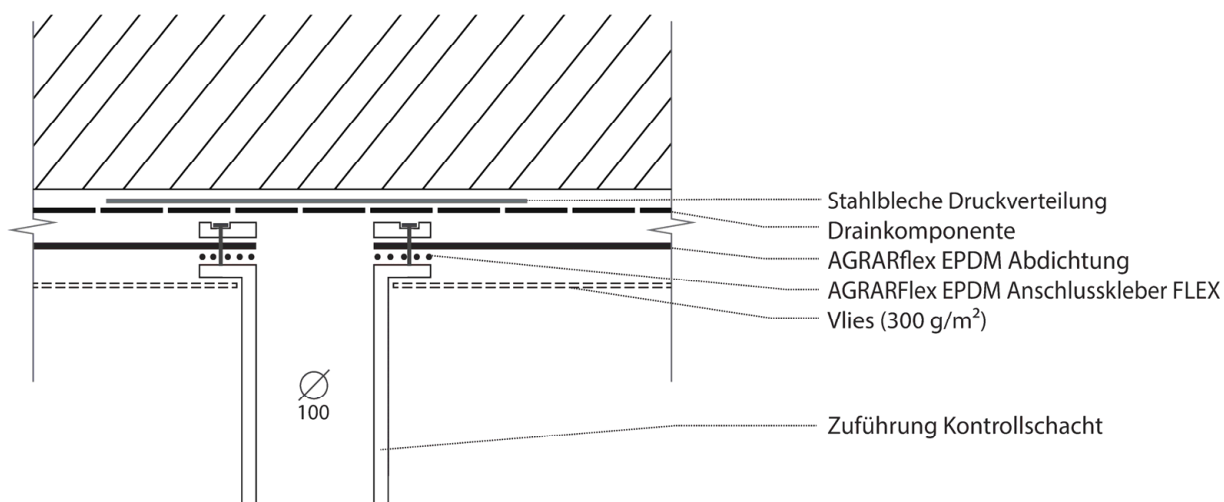
Abb. 2: Ausbildung Zuführung zum Kontrollschacht unterhalb der Bodenplatte
